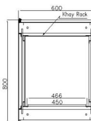
Mặt cắt 1-1
