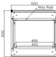
Mặt cắt 1-1
