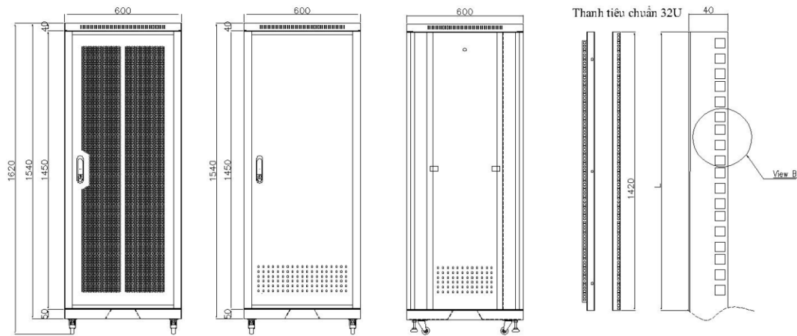
Mặt trước Rack
