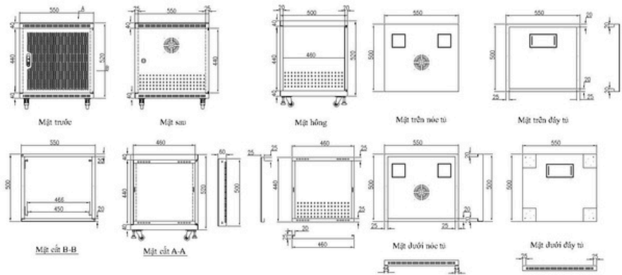
Bản vẽ tủ 9U D500
