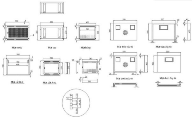
Bản vẽ tủ 6U D400 treo
