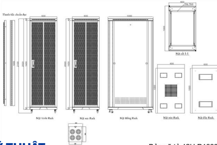
Bản vẽ tủ 42U D1000
