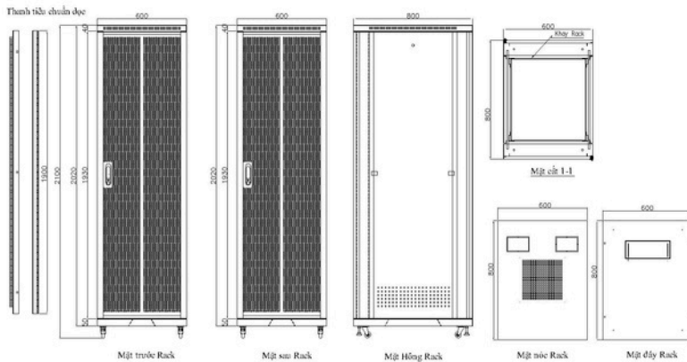
Bản vẽ tủ 42U D800
