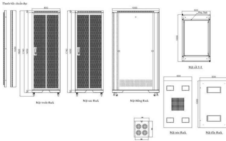
Bản vẽ tủ 36U D1000
