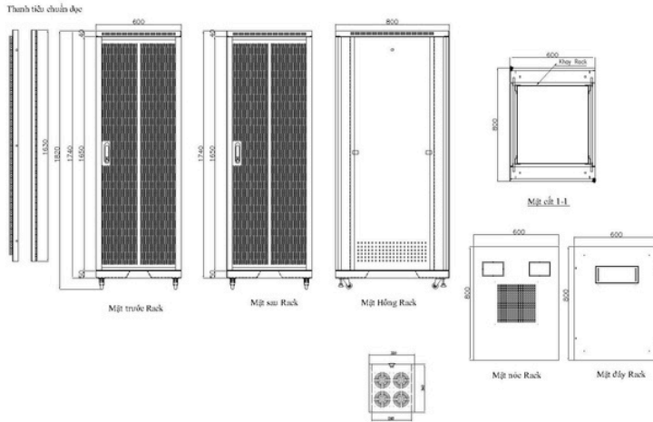
Bản vẽ tủ 36U D800
