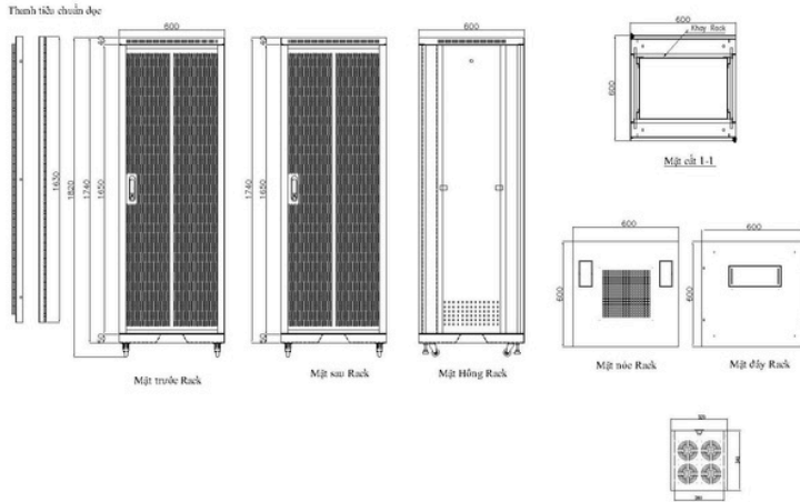
Bản vẽ tủ 36U D600
