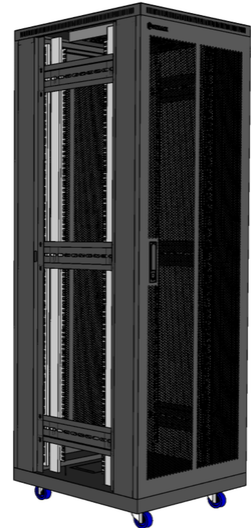
Bản vẽ tủ 36U D600
