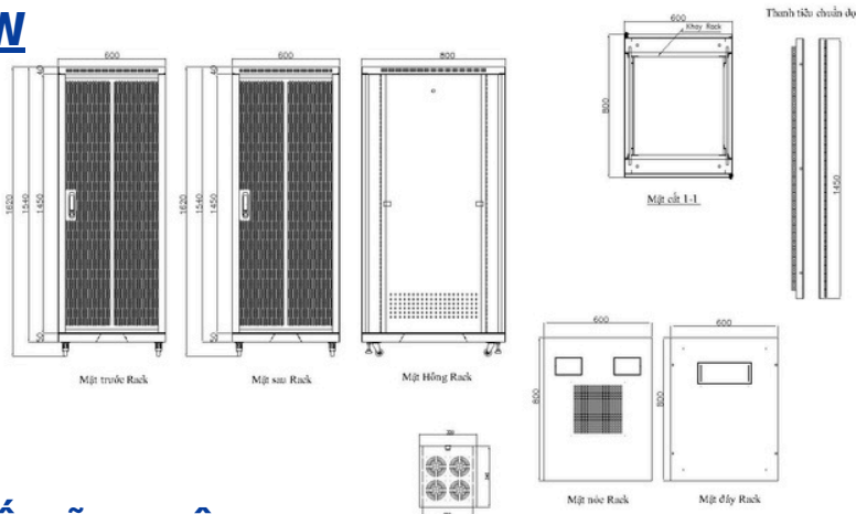
Bản vẽ tủ 32U D800
