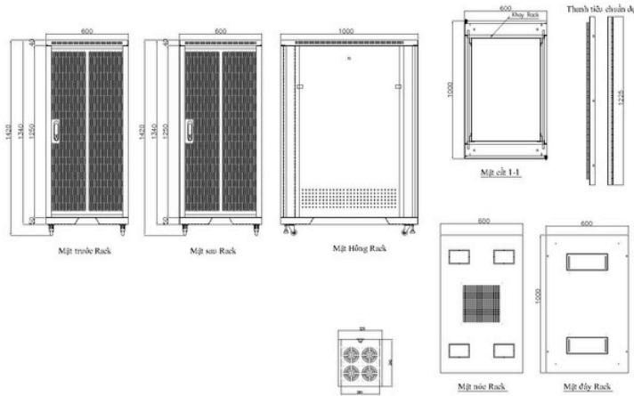
Bản vẽ tủ 27U D1000
