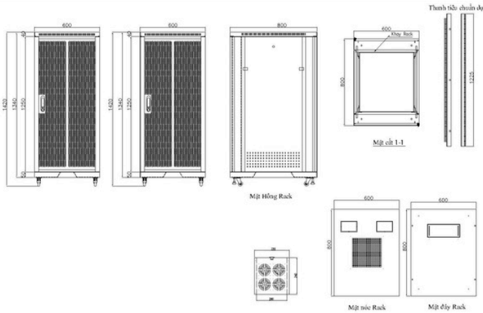
Bản vẽ tủ 27U D800
