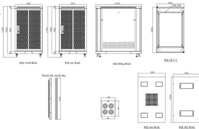
Bản vẽ tủ 20U D1000
