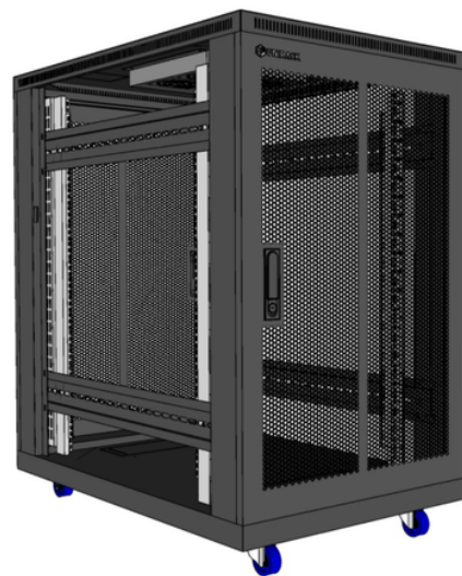
Bản vẽ tủ 20U D1000
