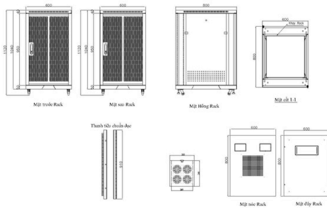
Bản vẽ tủ 20U D800
