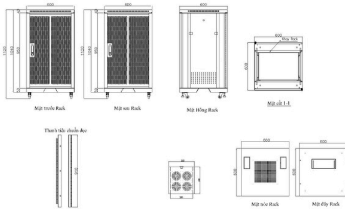
Bản vẽ tủ 20U D600
