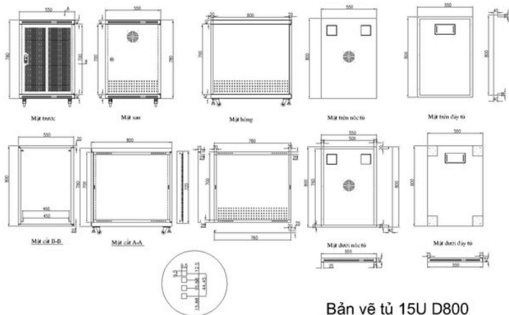
Bản vẽ tủ 15U D800
