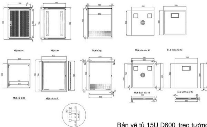
Bản vẽ tủ 15U D600 treo tường
