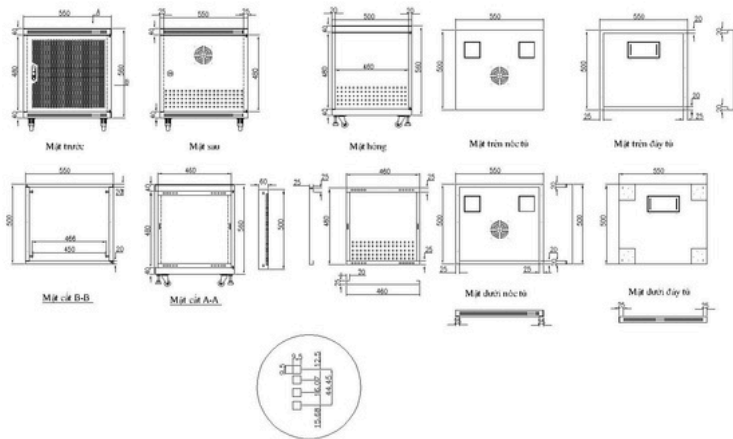
Bản vẽ tủ 10U D500
