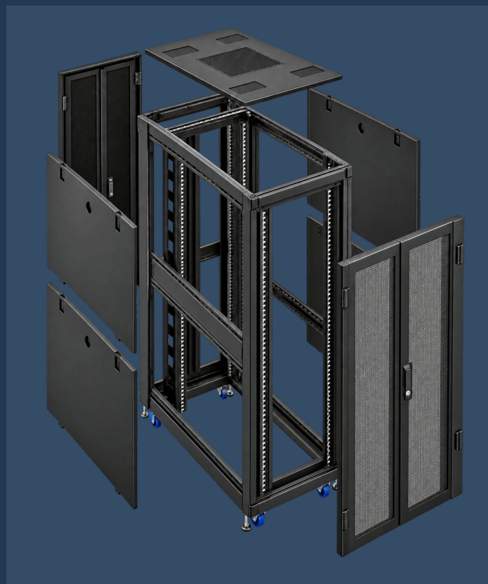
Bản tách rời cấu kiện
